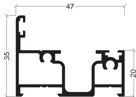
XP-24 Aro fixo guia de correr
