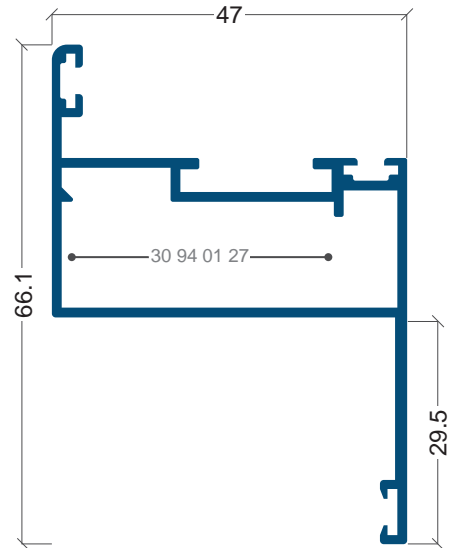
XP-26 Aro fixo com remate
