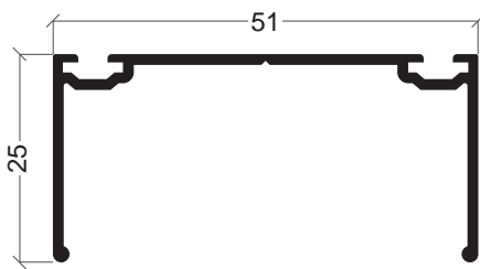
XP-20 Distanciador aro fixo de correr
